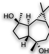
(-)-4β-7α-aromadendenediol
