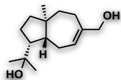
schisanwilsonene A
