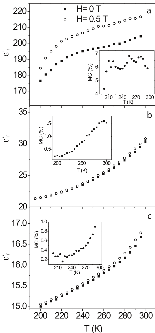
Fig. 8. Variación de la constante dieléctrica ( \epsilon' ) con la temperatura, e influencia de la aplicación de un campo magnético (H), para (a) Fe_3O_4 , (b) NiFe_2O_4 y (c) Fe_3O_4@SiO_2 , medidas a \nu = 3906 Hz. Detalle: Efecto magnetocapacitivo, donde MC = [\epsilon'_{r(H=0.5T)} - \epsilon'_{r(H=0T)}] / \epsilon'_{r(H=0T)} .
