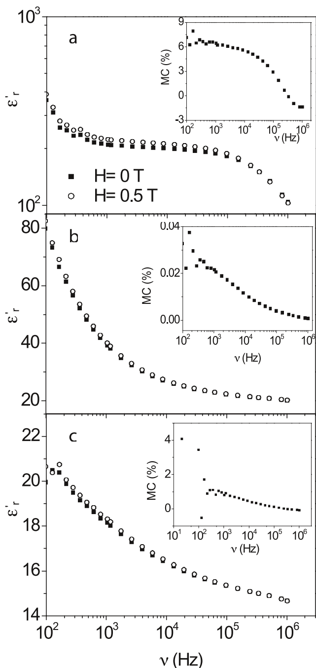
Fig. 7. Variación de la constante dieléctrica ( \epsilon' ) con la frecuencia ( \nu ) e influencia de la aplicación de un campo magnético (H), para (a) Fe_3O_4 , (b) NiFe_2O_4 y (c) Fe_3O_4@SiO_2 , medidas a T = 300 K. Detalle: Efecto magnetocapacitivo, donde MC = [\epsilon'_{r(H=0.5T)} - \epsilon'_{r(H=0T)}] / \epsilon'_{r(H=0T)} .
