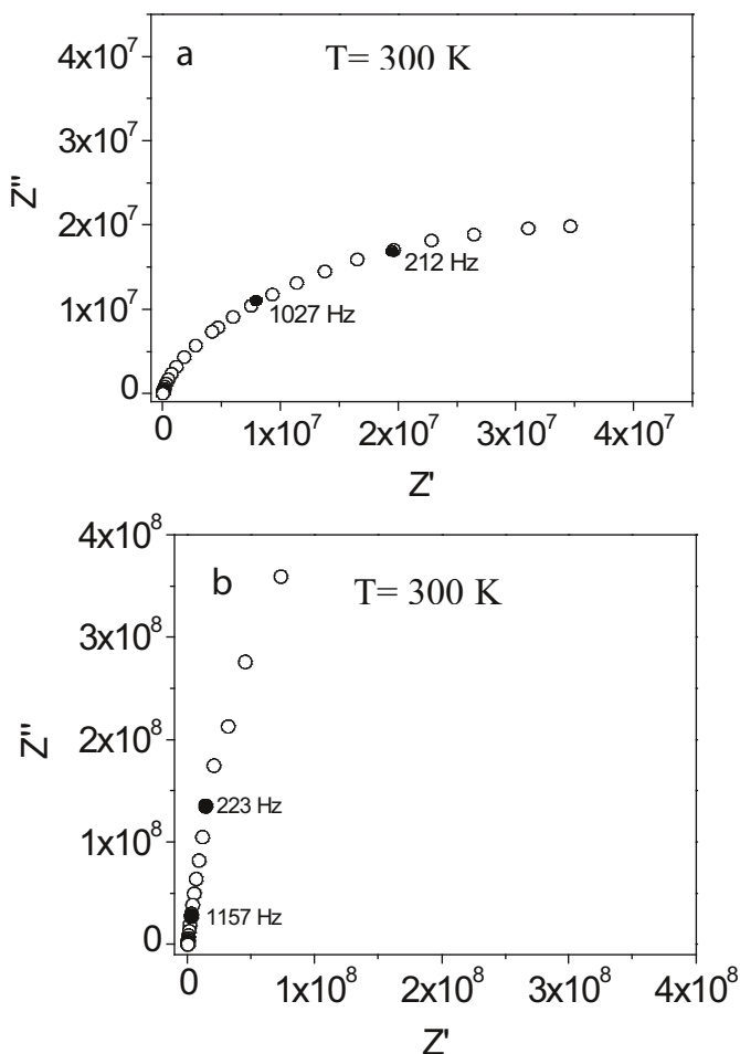
Fig. 6. Diagramas de impedancia compleja de (a) \text{NiFe}_2\text{O}_4 y (b) \text{Fe}_3\text{O}_4/\text{SiO}_2 , a 300 K. Estos comportamientos son representativos para todo el intervalo de temperaturas estudiado.
