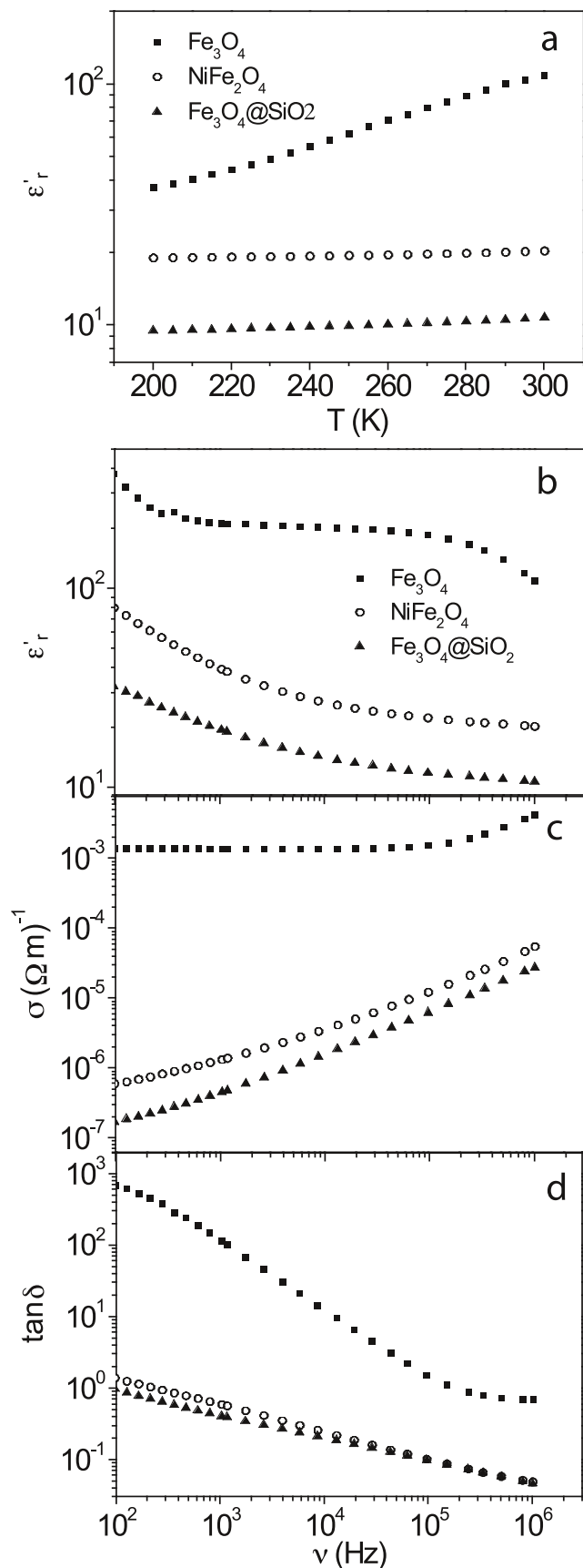
Fig. 4. (a) Variación de la constante dieléctrica en función de la temperatura, medida a \nu = 1 MHz para las tres muestras. Variación de: (b) la constante dieléctrica ( \epsilon' ), (c) la conductividad ( \sigma_{ac} ) y (d) la tangente de pérdidas ( \tan \alpha ), en función de la frecuencia, medida a T = 300 K para las tres muestras.
