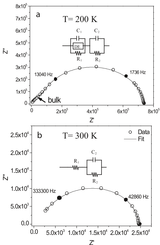
Fig. 5. Diagramas de impedancia compleja de la muestra \text{Fe}_3\text{O}_4 y sus correspondientes ajustes a (a) 200 K, y (b) 300 K. La figura 5(a) es representativa del comportamiento a 200 \leq T(\text{K}) \leq 225 , y la 5(b) del comportamiento a 225 < T(\text{K}) \leq 300 . Los círculos representan los datos experimentales y las líneas representan los correspondientes ajustes.
